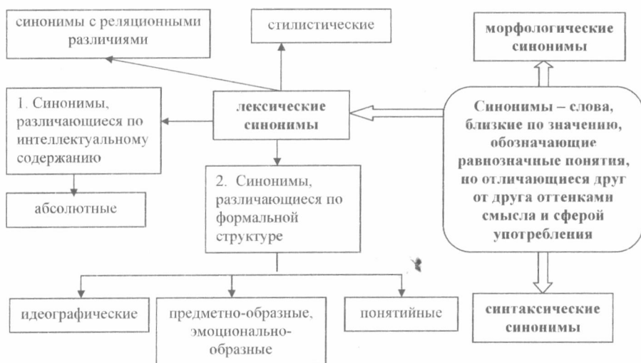
Рис.11 – Классификация синонимов
