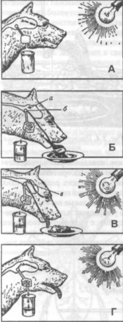
Рис. 3.6. Образование условного рефлекса у животных (по И. П. Павлову). Объяснения в
