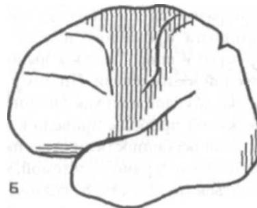
Рис. 4.2. Кора мозга обезьяны (А) и человека (Б). Заштрихованные участки — проекционные поля. Незаштрихованные участки — интегративные поля. У человека площадь интегративных полей значительно больше.
