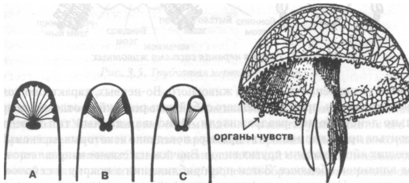
Рис. 3.2. Дифференциация органов чувств у животных на стадии элементарного поведения.
