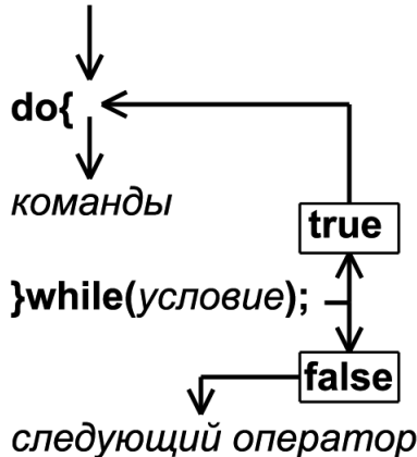
Рис. 4.10. Алгоритм выполнения оператора do-while
