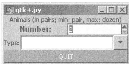
PyGTK
