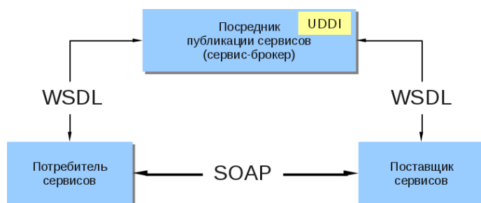
Рис. 5.1. Концепция веб-сервиса
