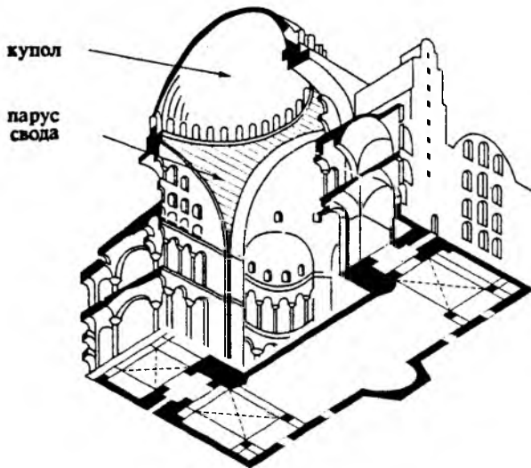
Храм крестово-купольного типа
